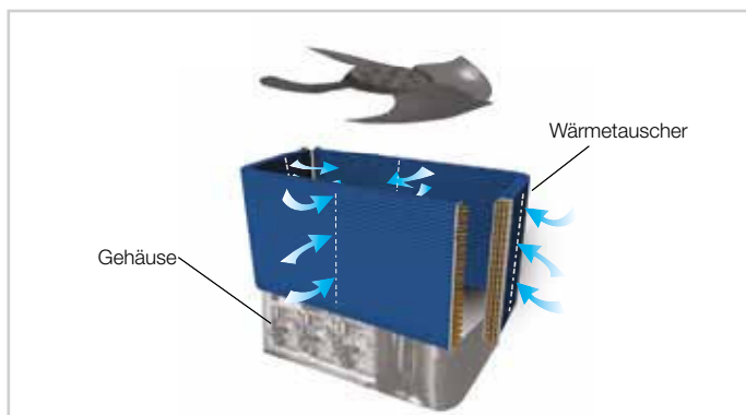
4-seitiger Wärmetauscher erzielt einen ausgewogenen Luftstrom
