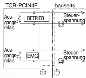
* Einbau der optionalen PCBs in Steuerungsbox der Haupt-Außengeräte.
