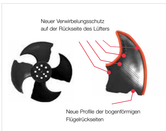
Fortschrittliche Schaufelformen für ein besseres Luftmanagement
