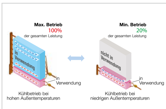
Variabler Wärmetauscher
